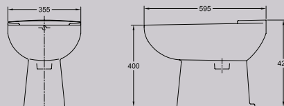
Deluxe bidet
