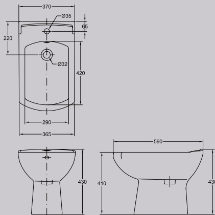
Zeto bidet
