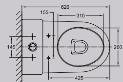
Deluxe bidet
