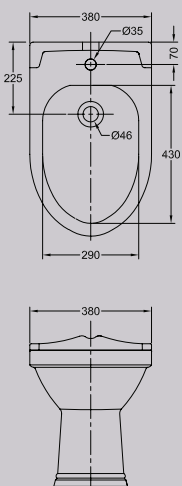
Carlton bidet
